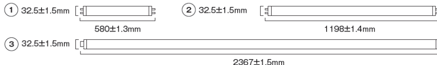
【FORCE BRIGHT 蛍光灯タイプ LED スペック表】
